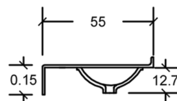
VISTA CORTE
